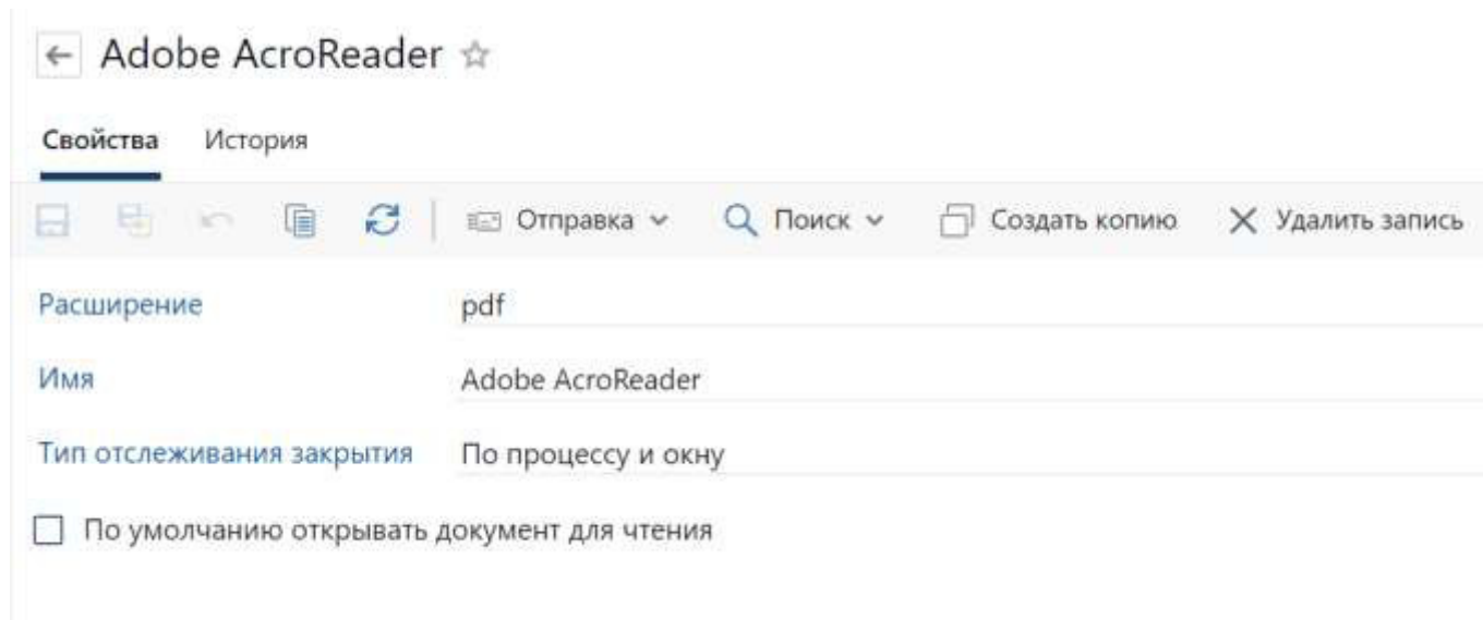
Рисунок 5.43 Создание приложения-обработчика
