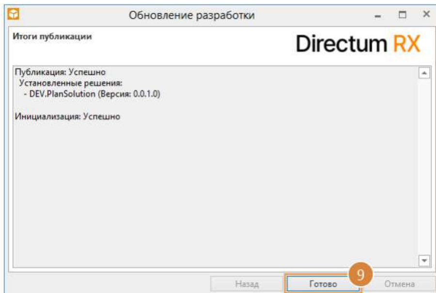
Рисунок 3.4 Завершение установки
